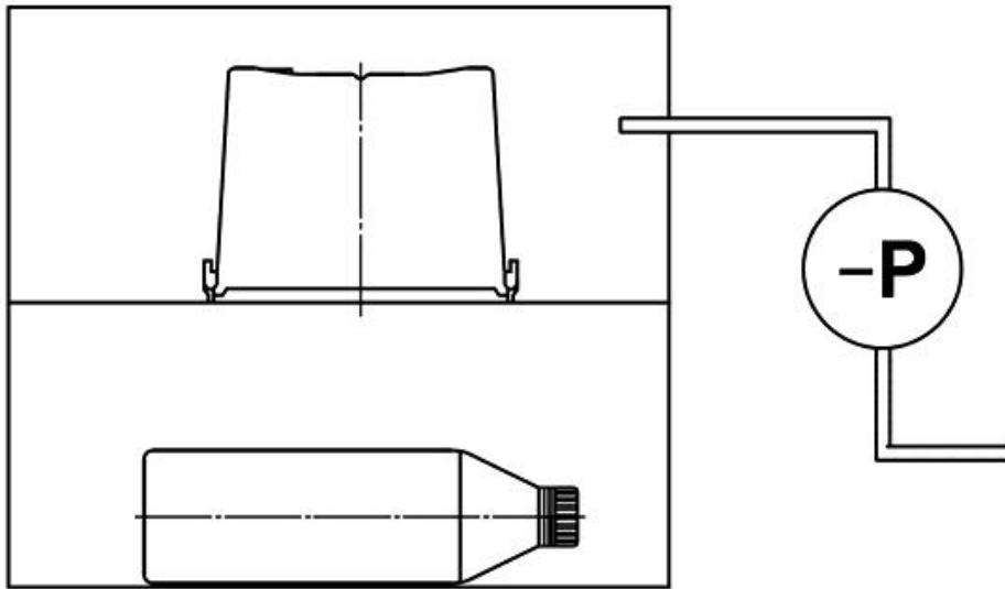
Рисунок 1 - Контроль герметичности упаковки в вакуумной камере
